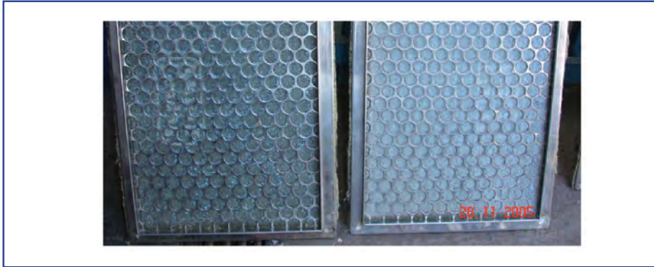
شکل ۷- تجمع ذرات بر روی سطح فیلتر کثیف (سمت چپ) و مقایسه با فیلتر تمیز (سمت راست)
